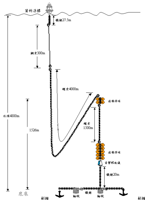
圖5 深海資料浮標錨繫設計
