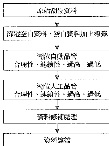
圖 1 潮位資料品管處理流程
