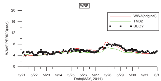
圖5 修正前後的周期與實測周期比較時序列圖-以WRF風場模擬波浪
