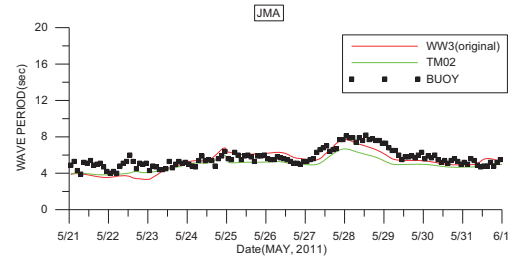
圖3 修正前後的周期與實測周期比較時序列圖-以JMA風場模擬波浪
